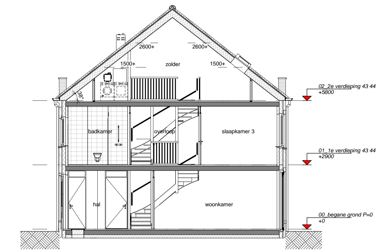
doorsnede B-B
