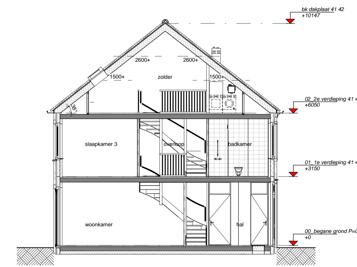
doorsnede A-A
