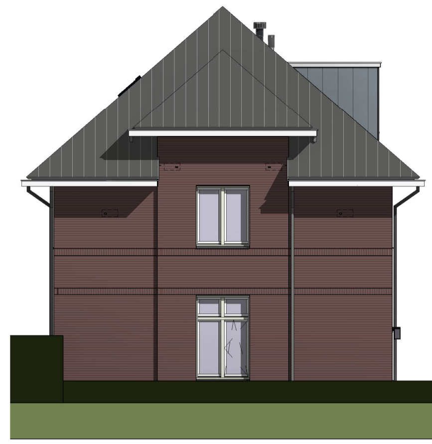
Linker zijgevel
