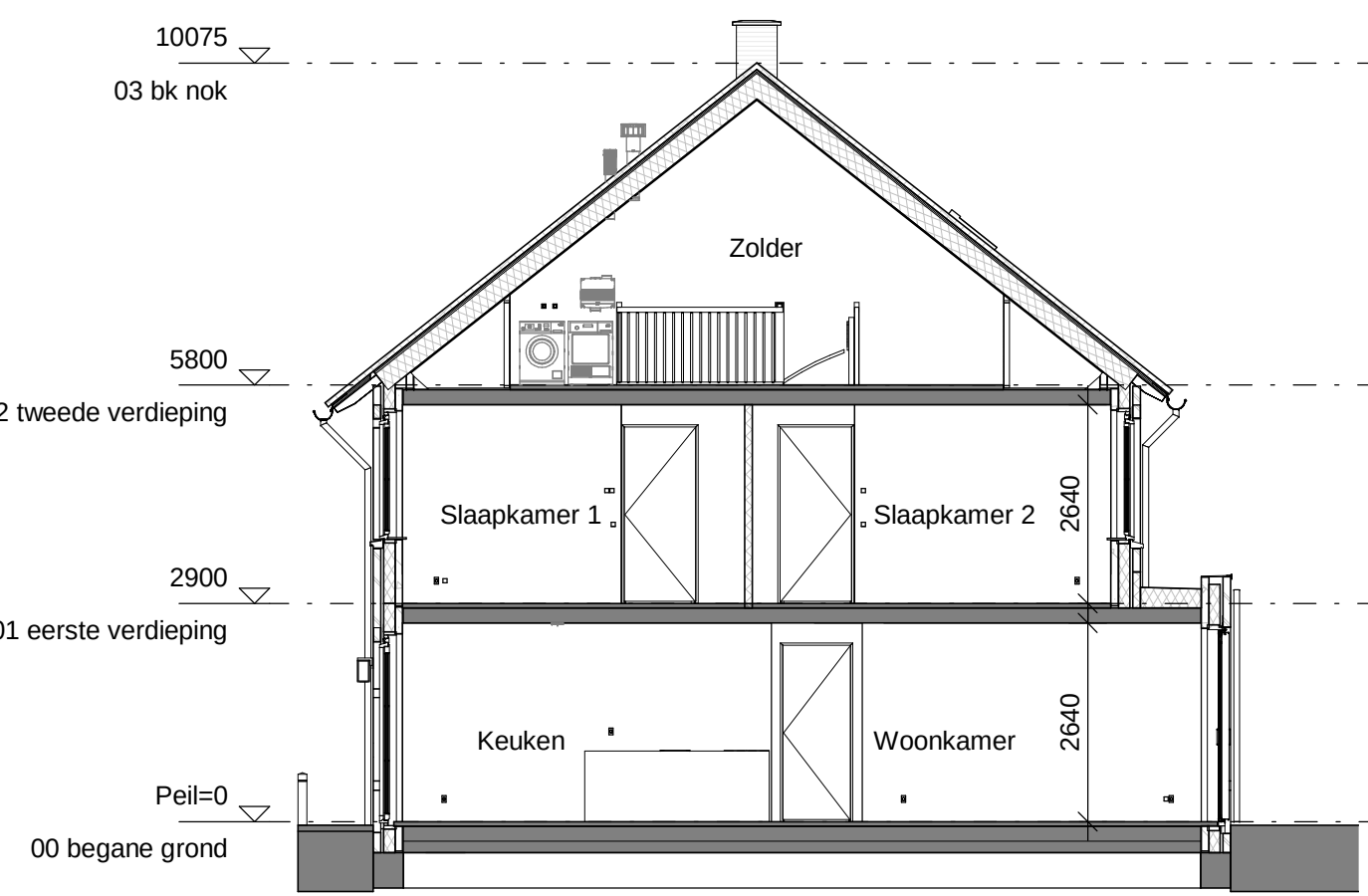
Doorsnede B
