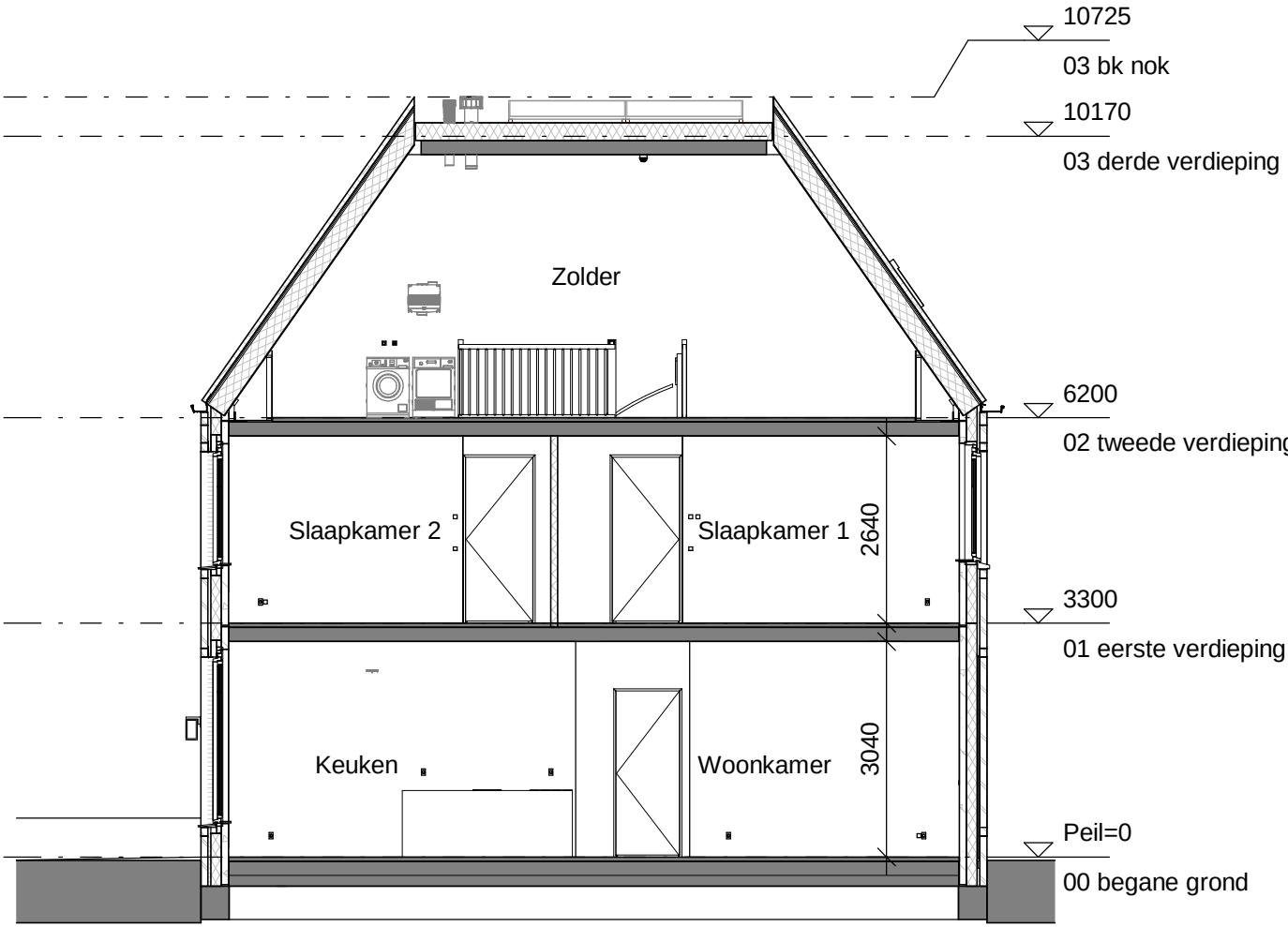
Doorsnede A
