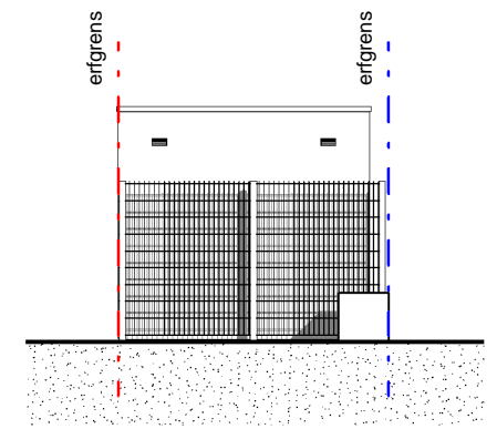
Rechter zijgevel schaal 1 : 100
