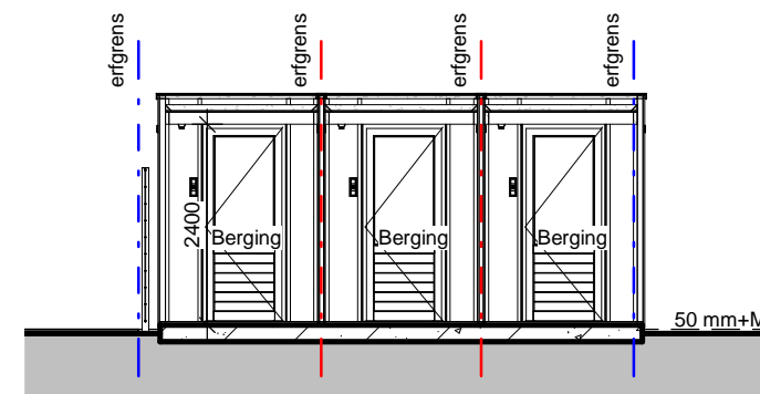
Doorsnede B1 schaal 1 : 100
