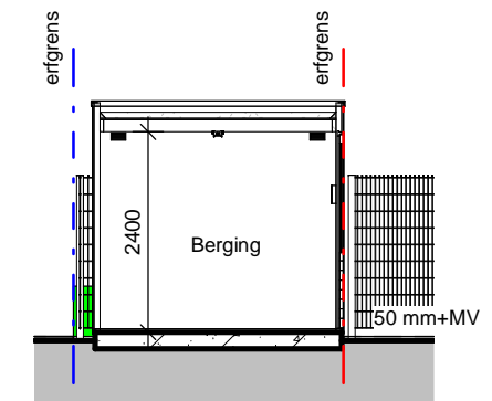
Doorsnede B2 schaal 1 : 100
