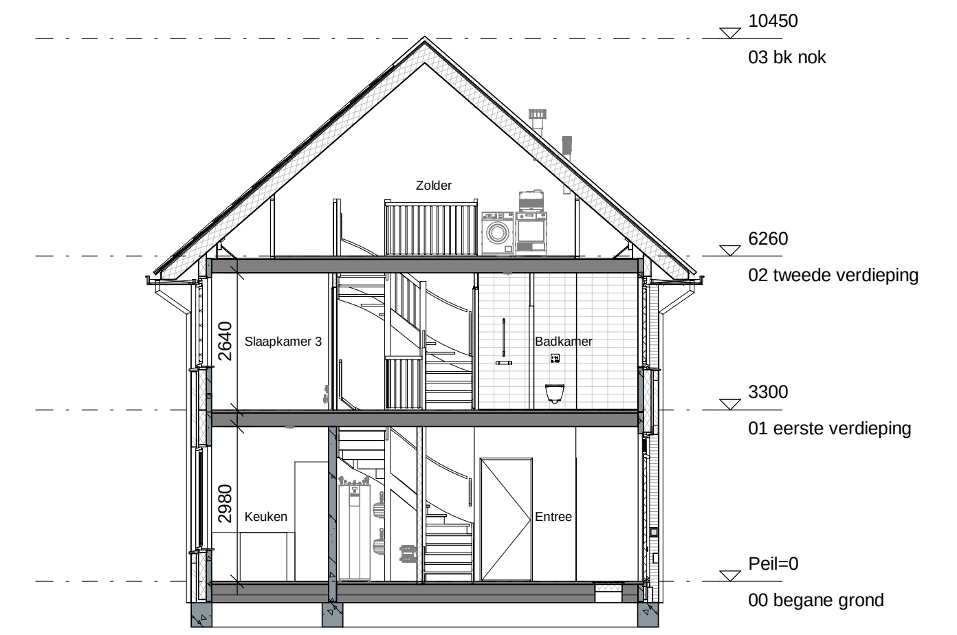
Doorsnede A
