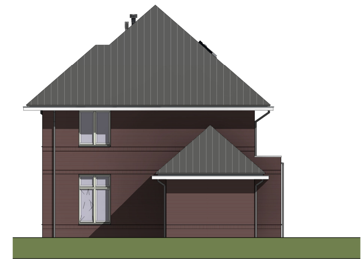
Rechter zijgevel
