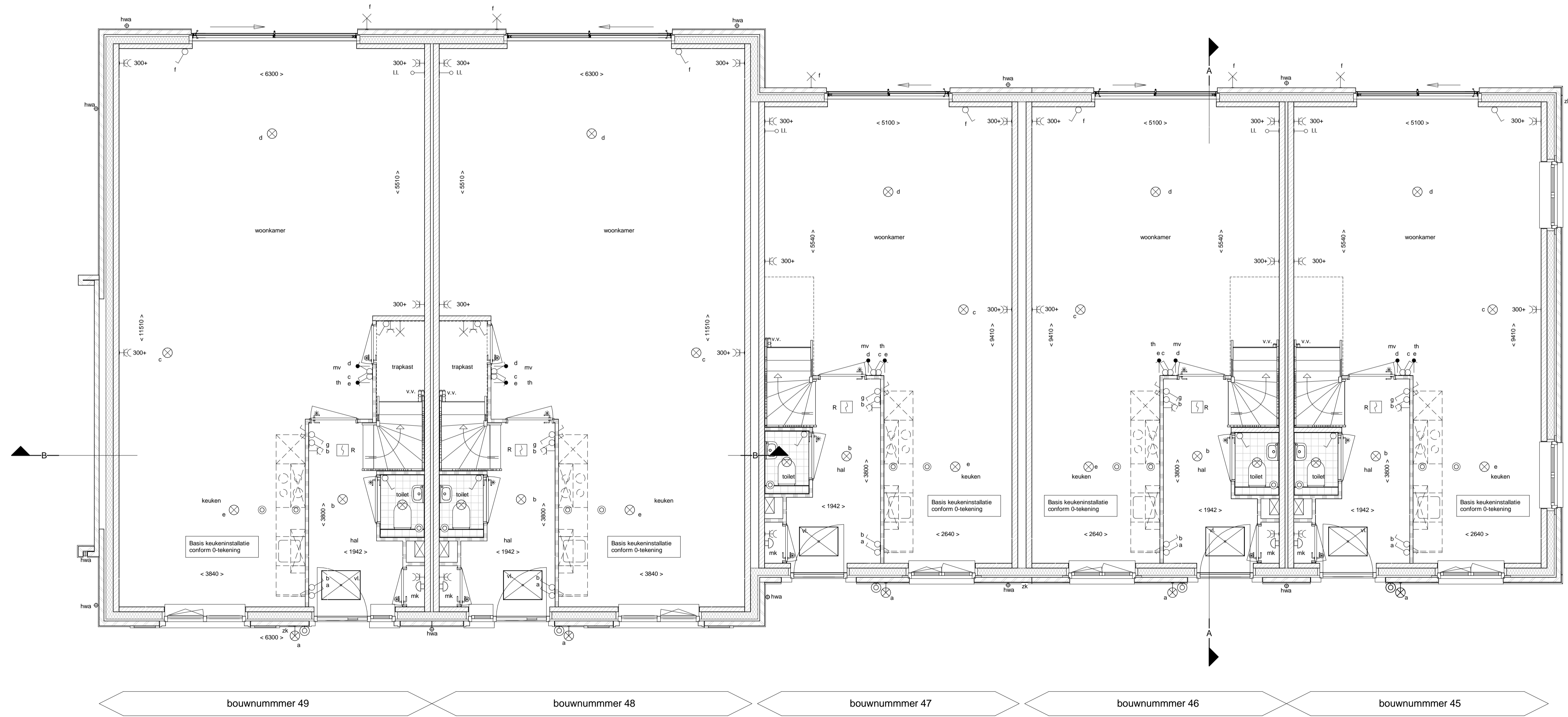
Beganegrond schaal 1 : 50
