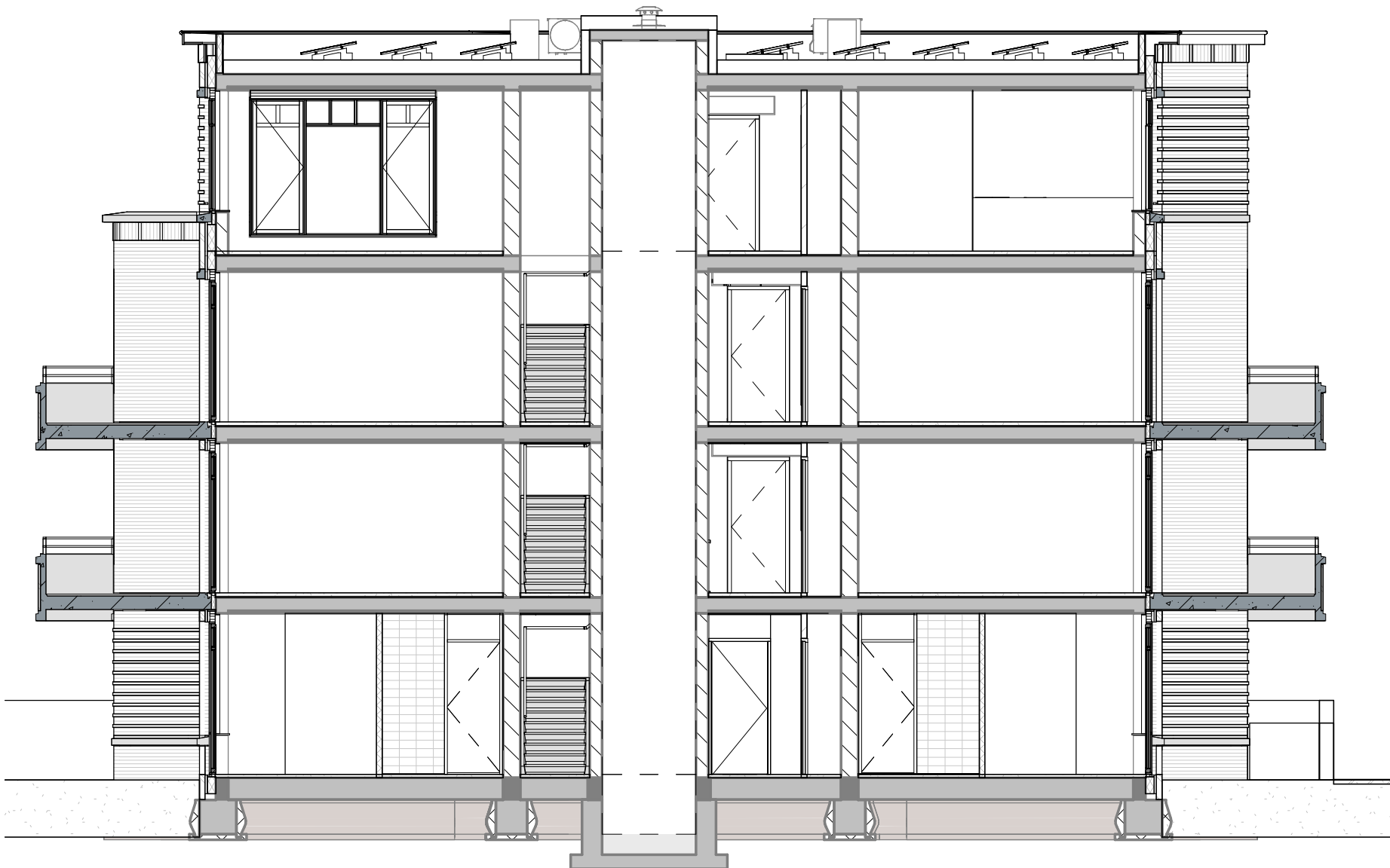
Doorsnede 02-B
