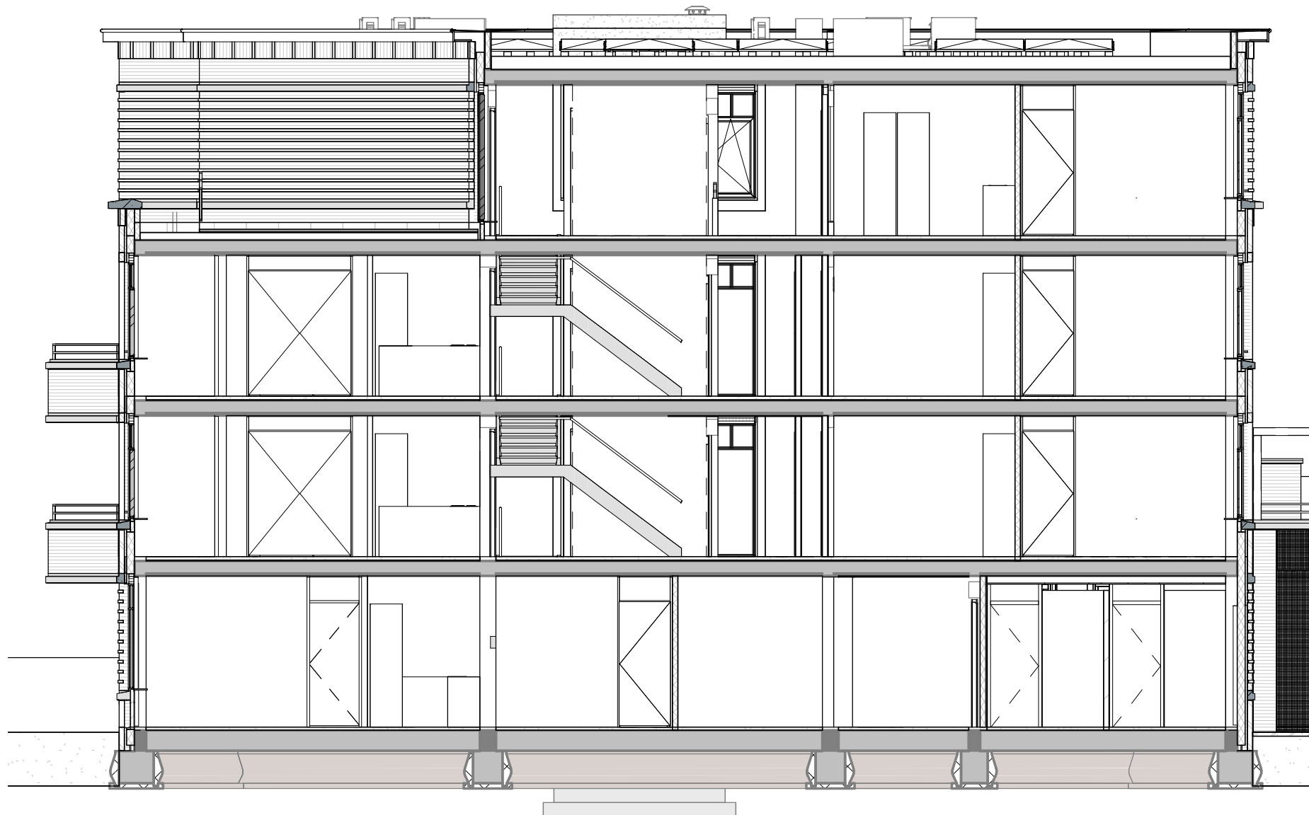
Doorsnede 02-A
