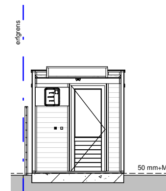
Doorsnede A-2
