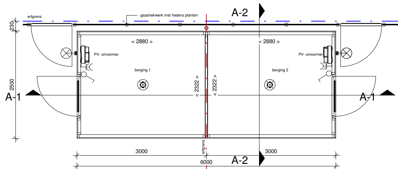
Begane grond
