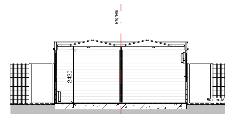
Doorsnede A-1
