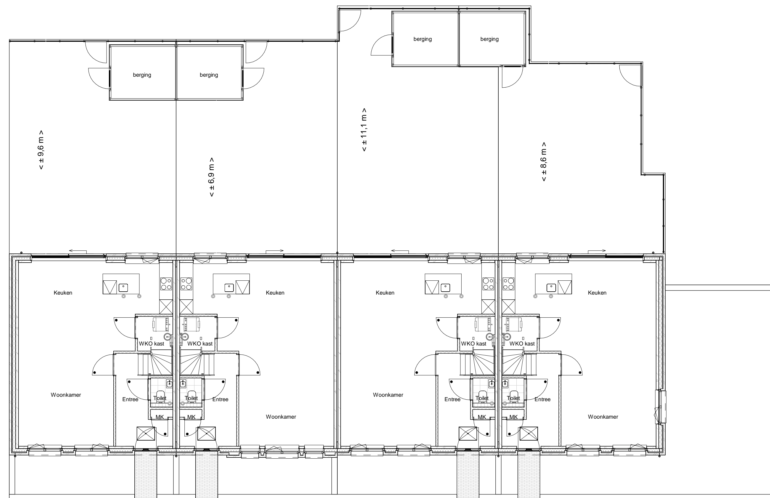
Begane grond
