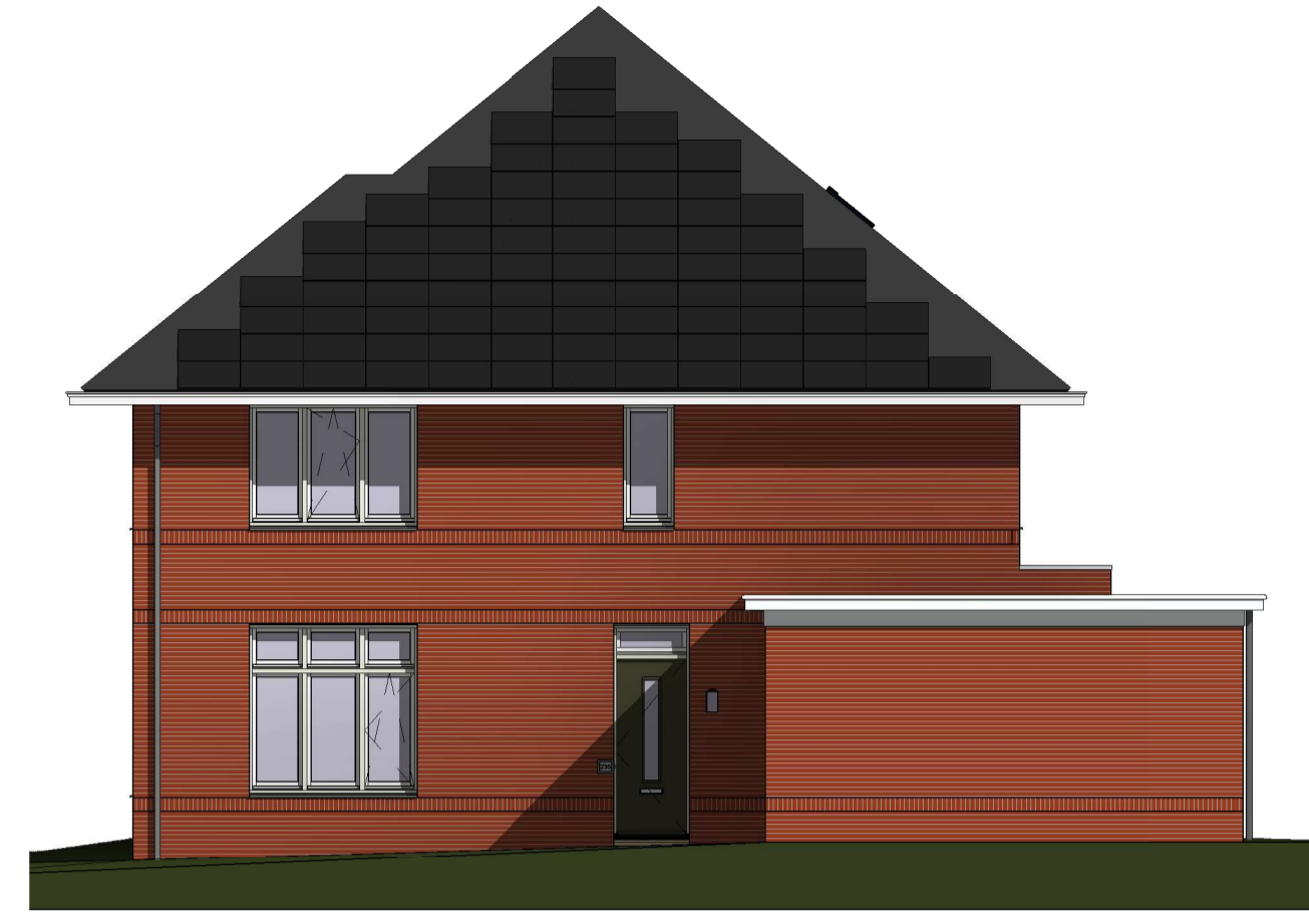
BN235 Rechter zijgevel
