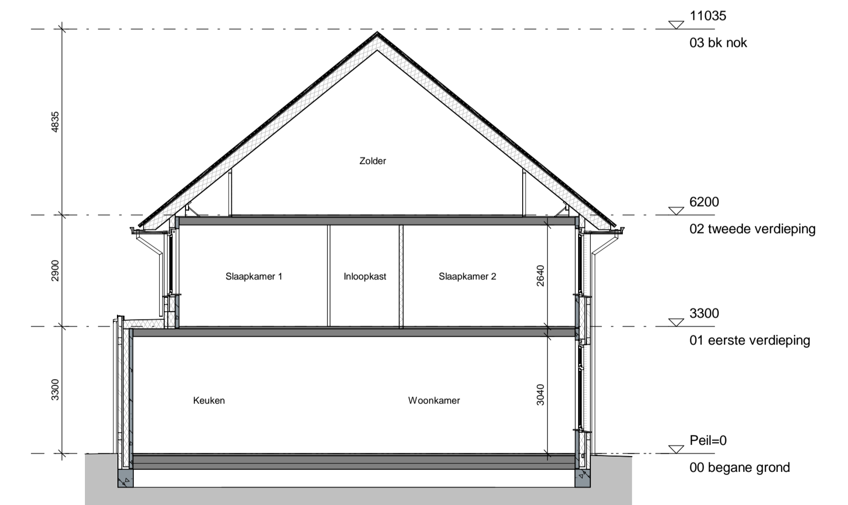
BN236 Doorsnede A
