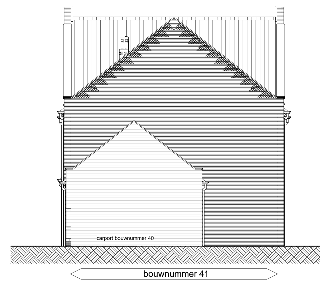
Rechterzijgevel schaal 1 : 100
