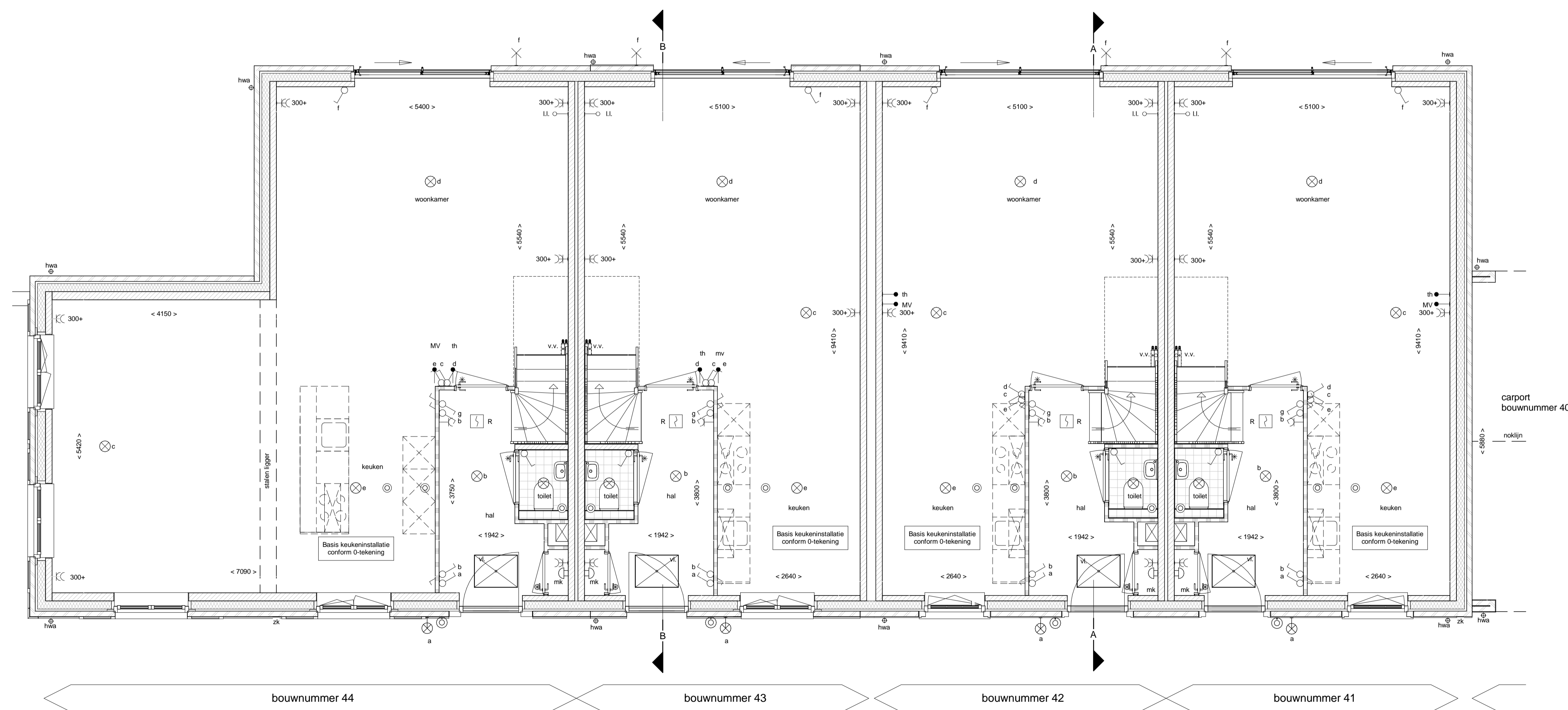
Begane grond schaal 1 : 50
