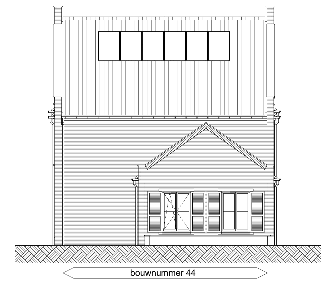
Linkerzijgevel schaal 1 : 100
