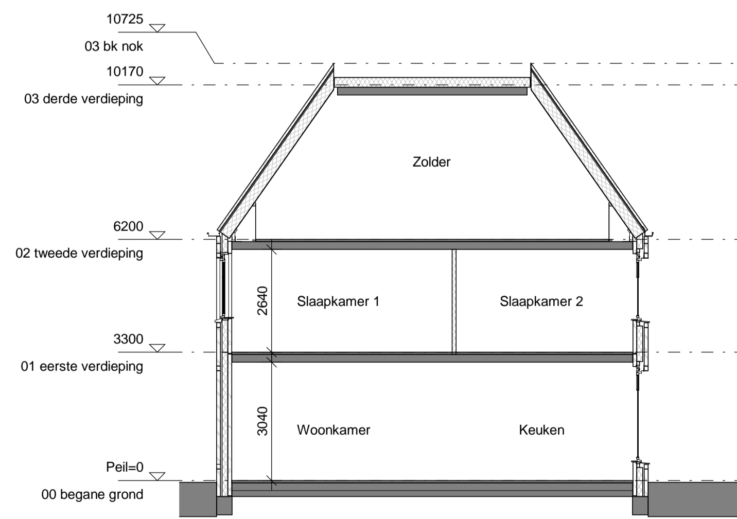
Doorsnede A
