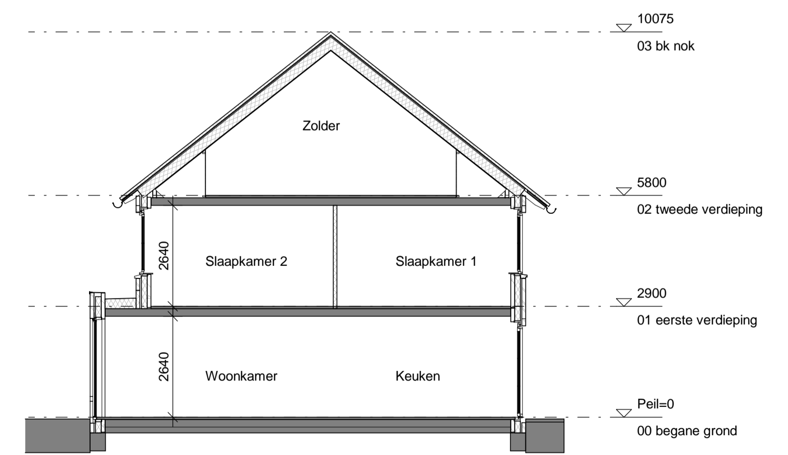
Doorsnede B
