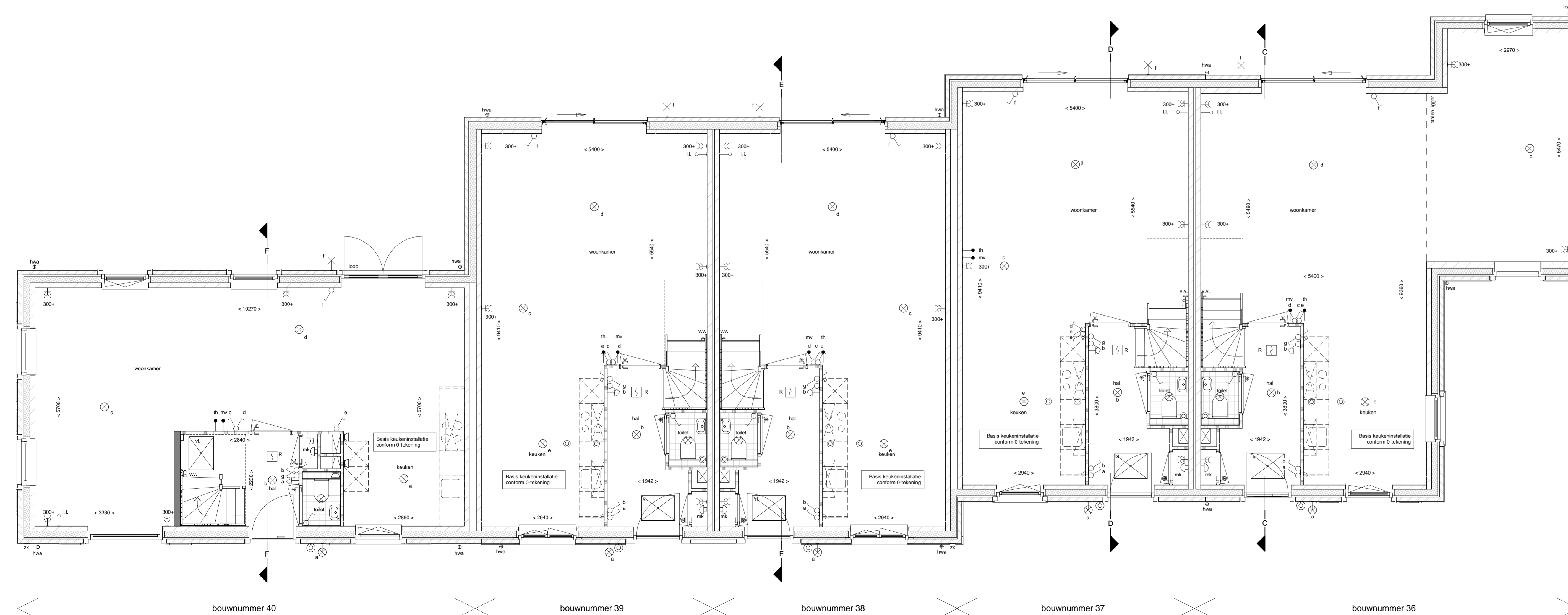
Beganegrand schaal 1 : 50
