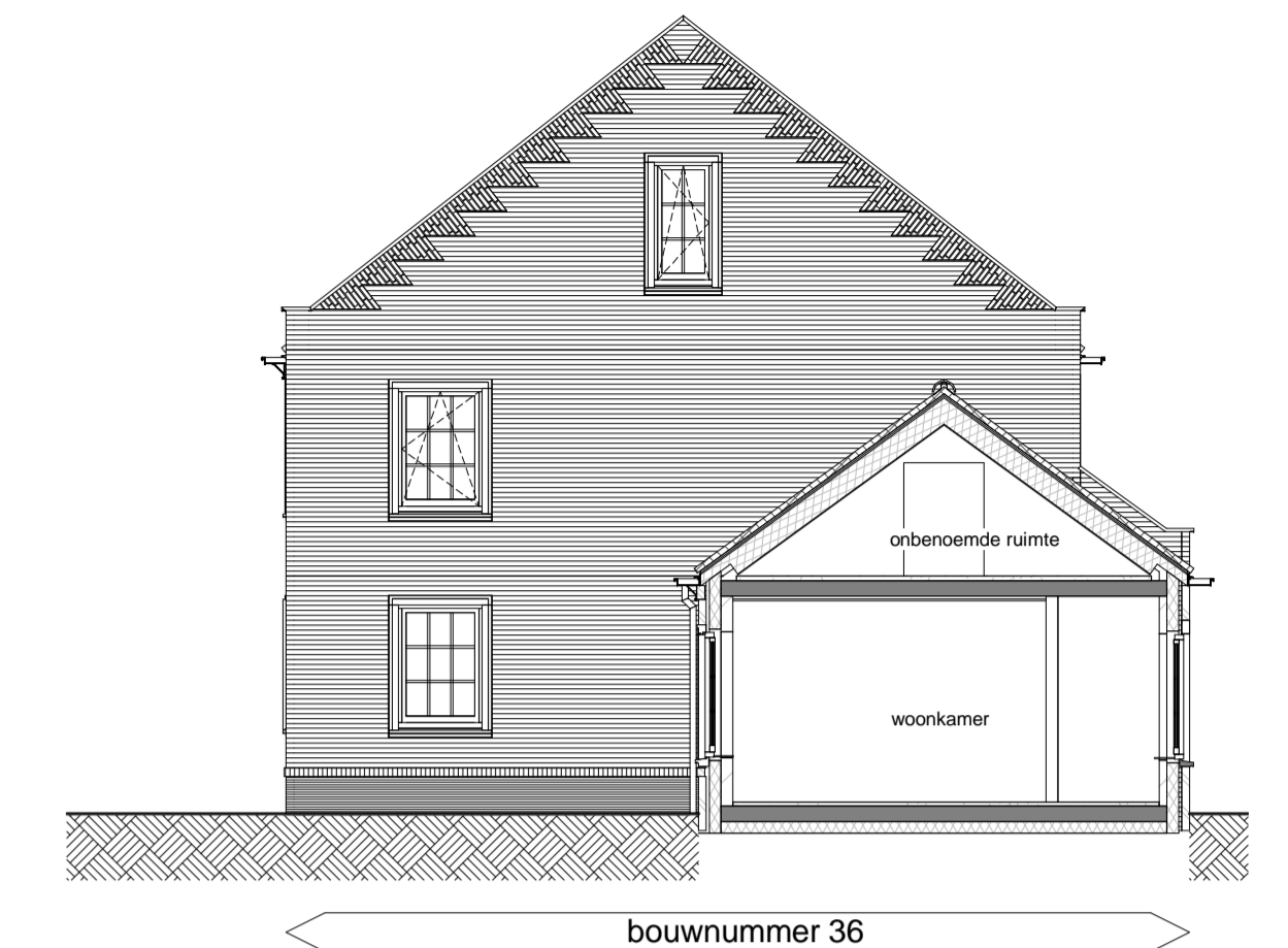
Rechterzijgevel schaal 1 : 100
