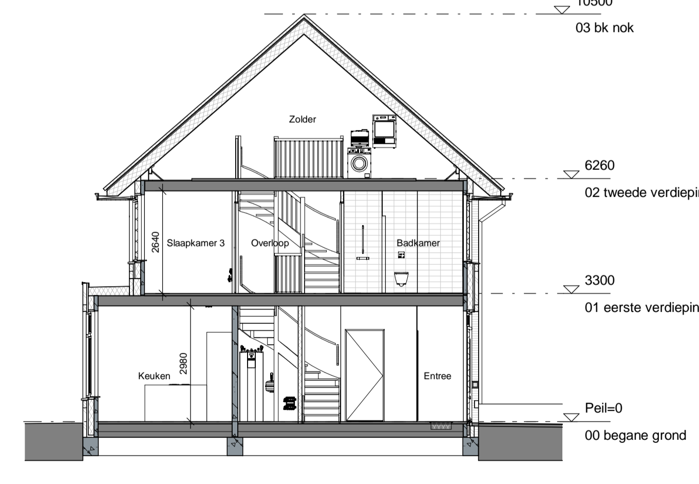
Doorsnede A
