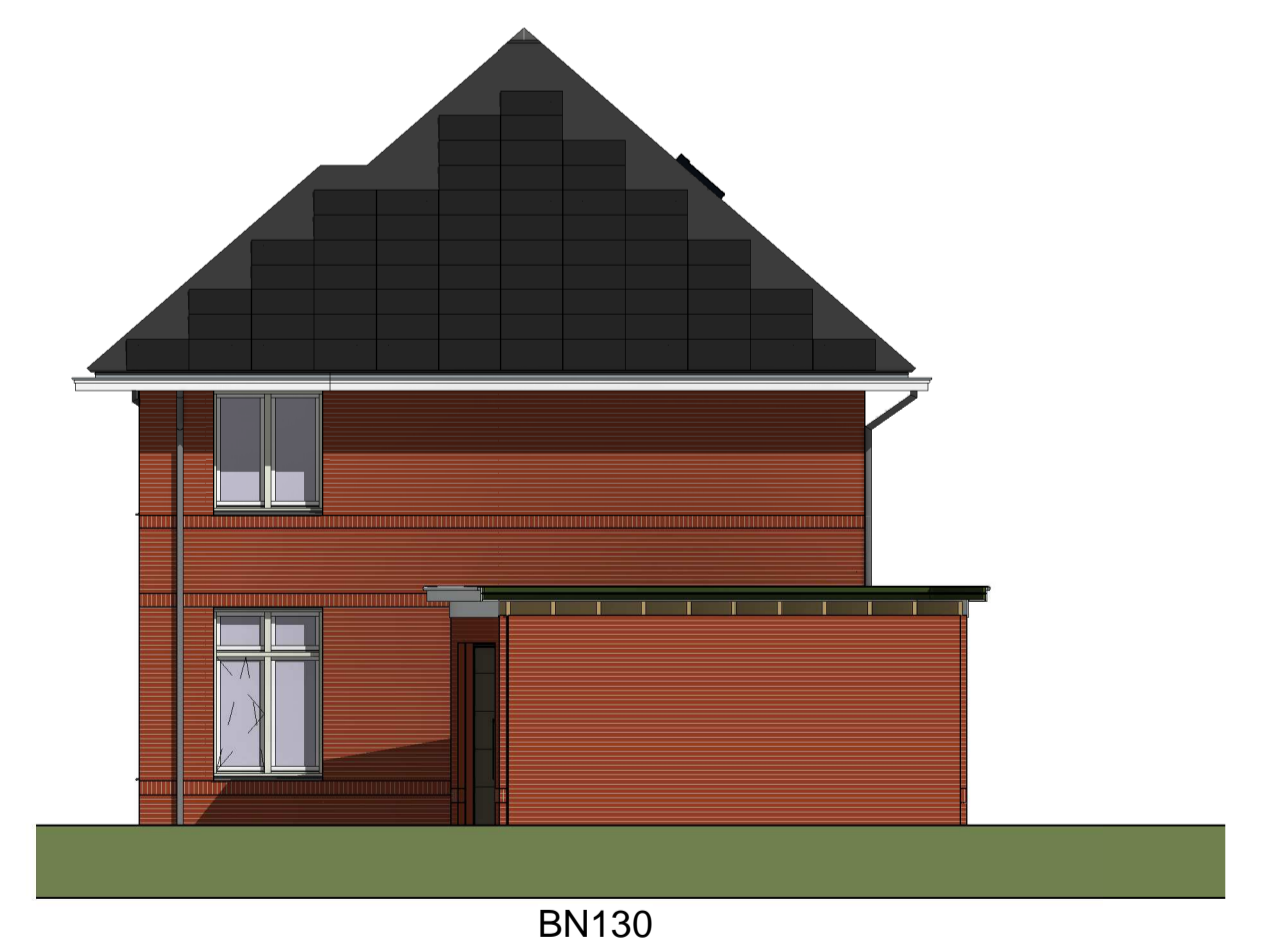
Rechter zijgevel
