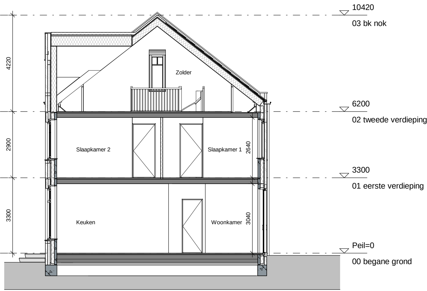
Doorsnede B
