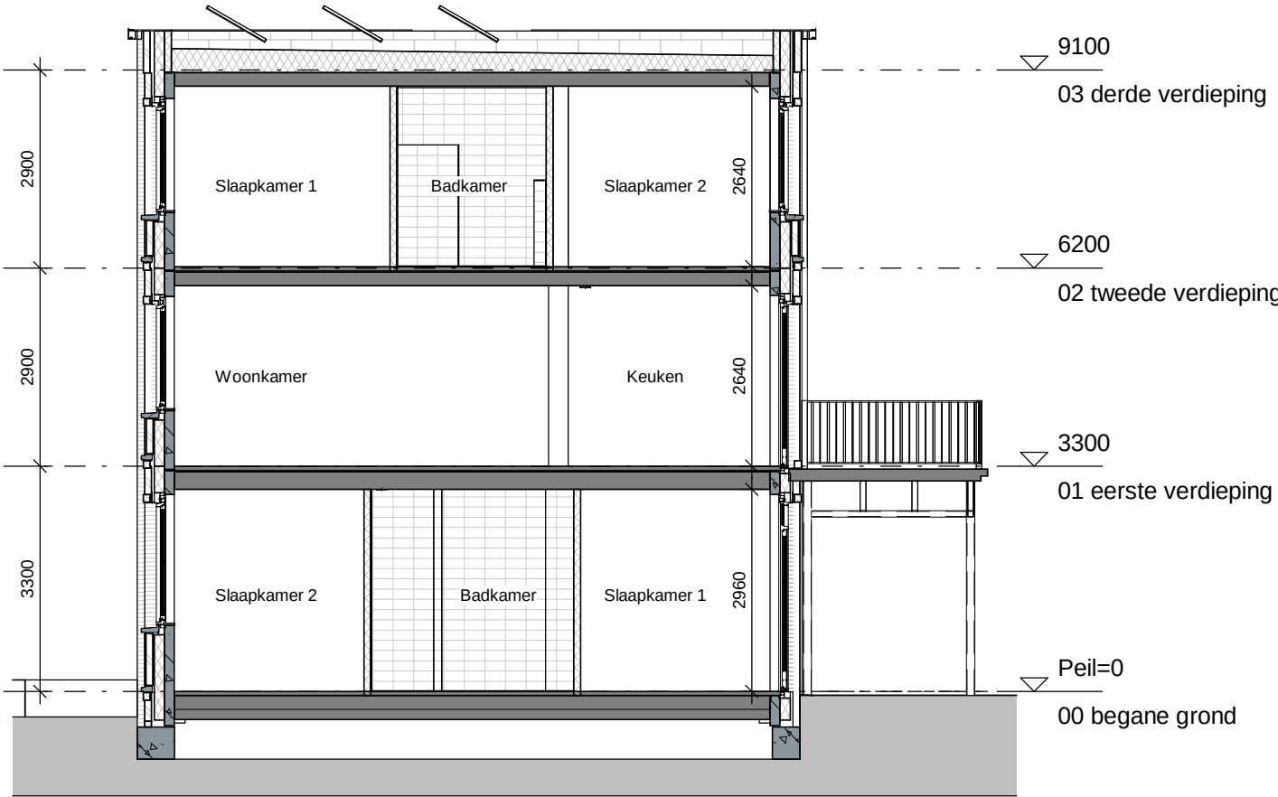
Doorsnede A
