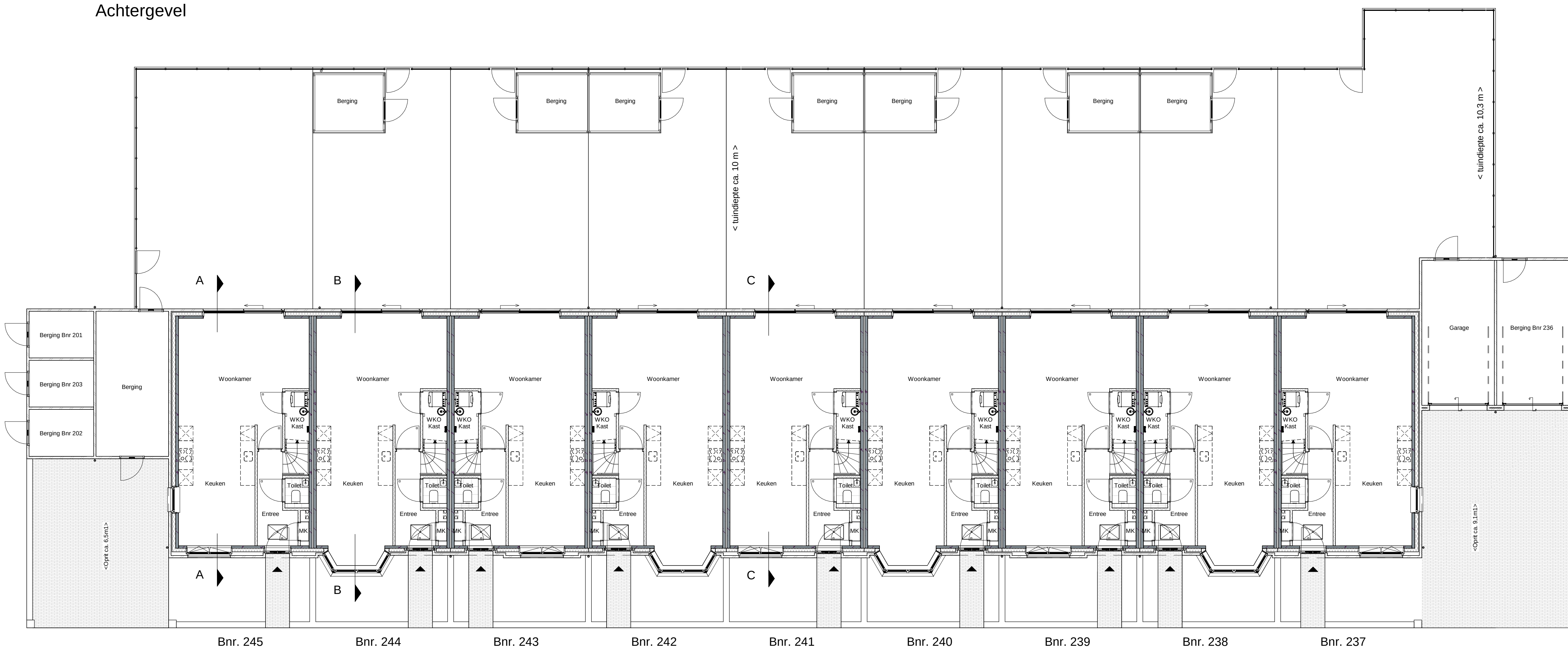
Begane grond
