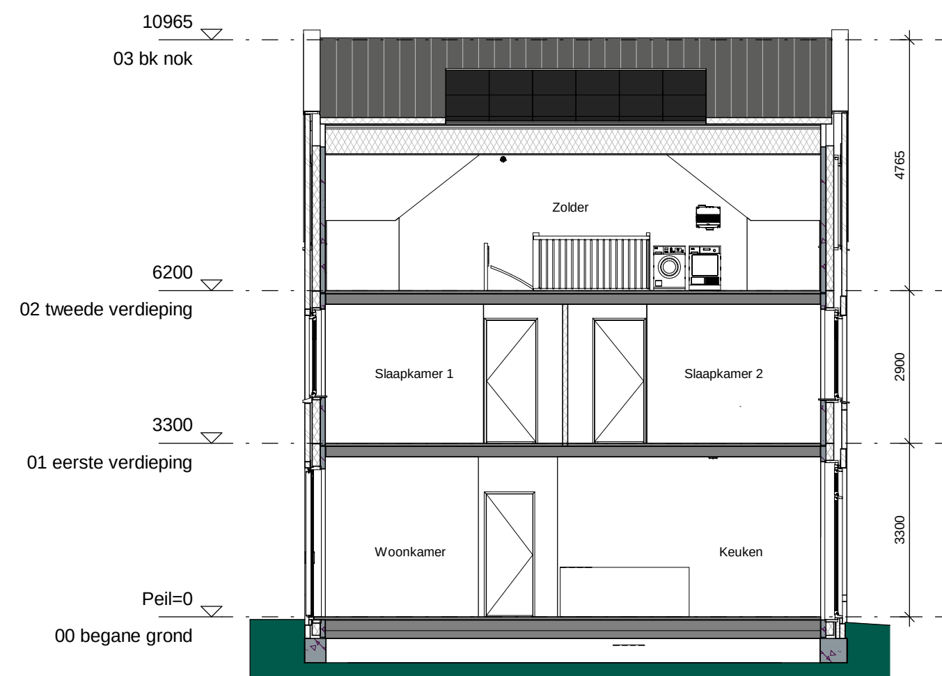
Doorsnede A
