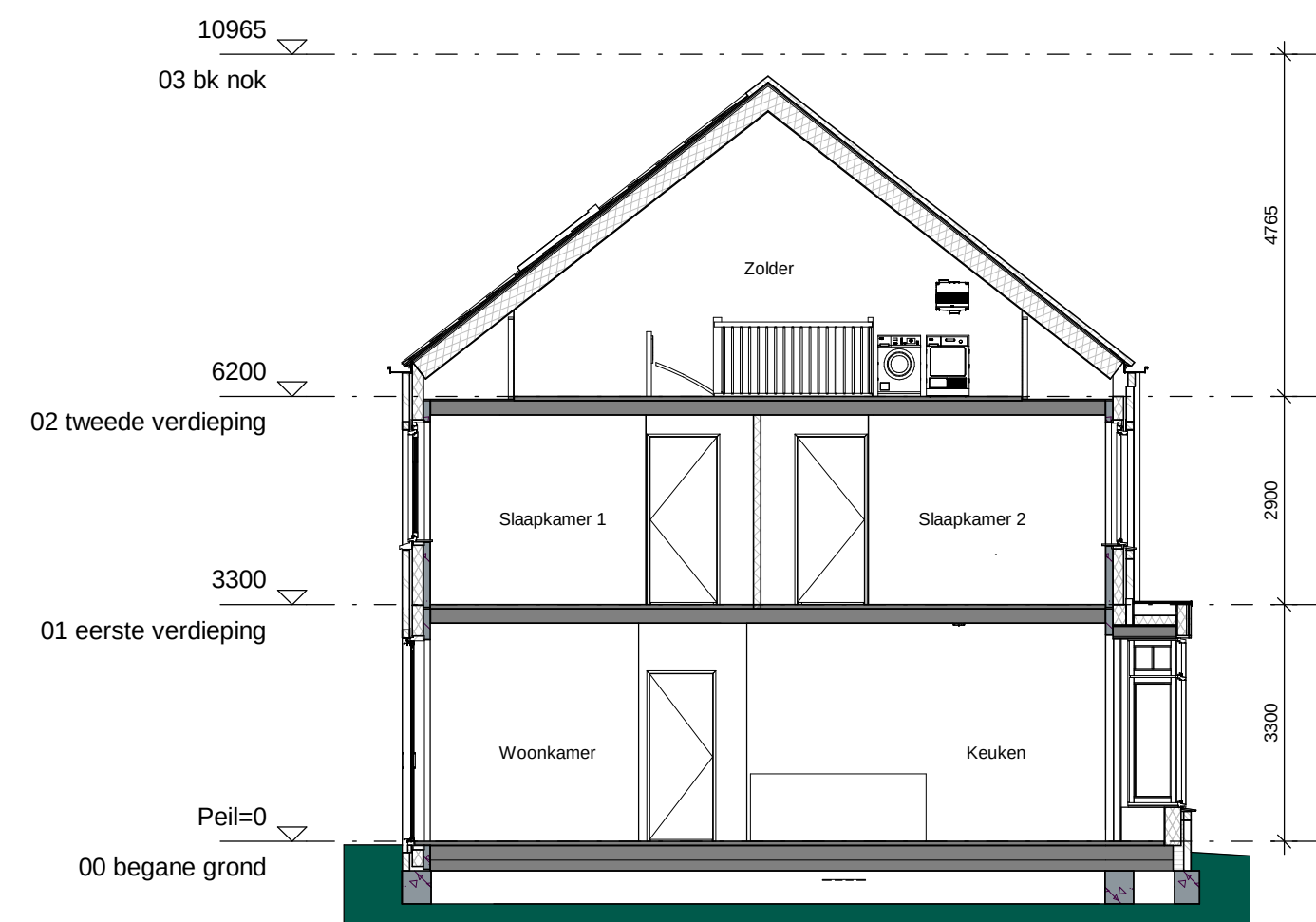
Doorsnede B
