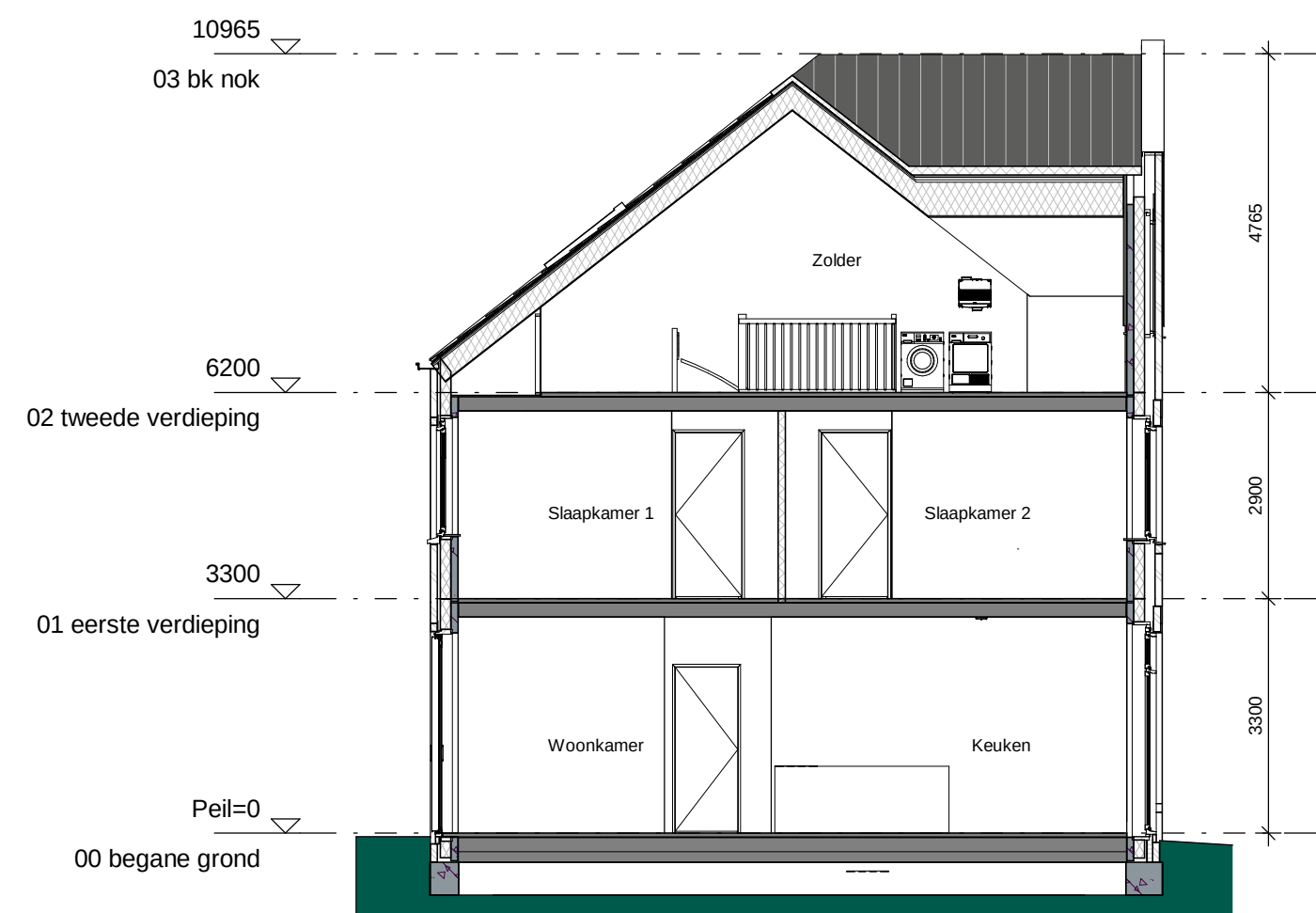
Doorsnede C
