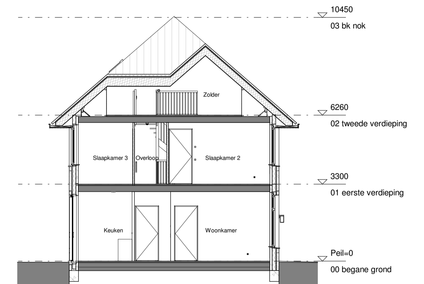
Doorsnede A
