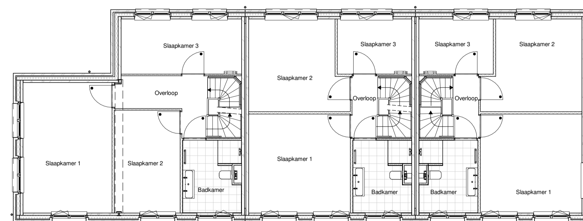
1e Verdieping
