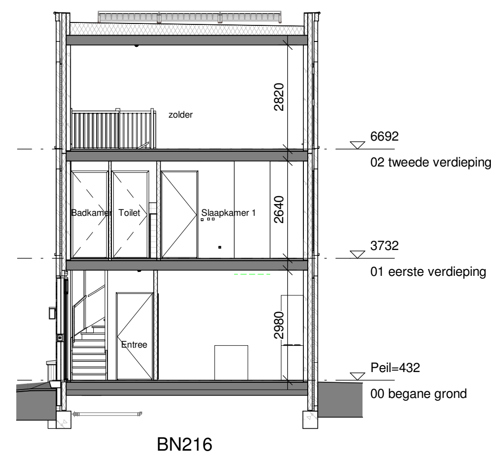
Doorsnede A
