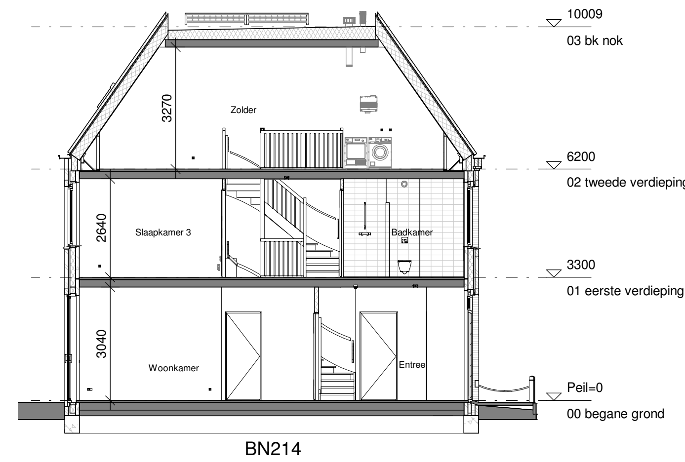
Doorsnede B
