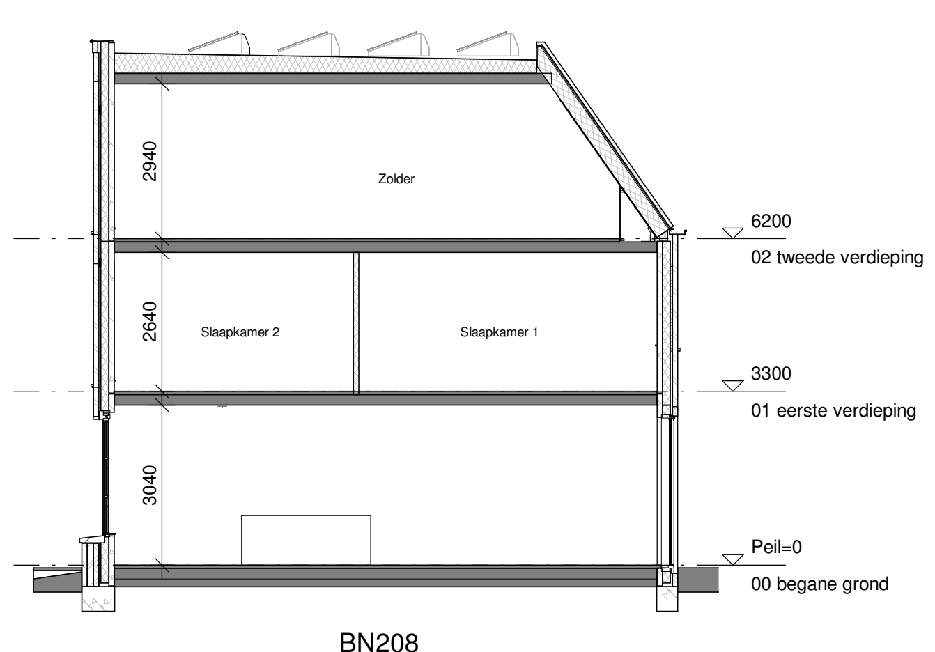
Doorsnede C
