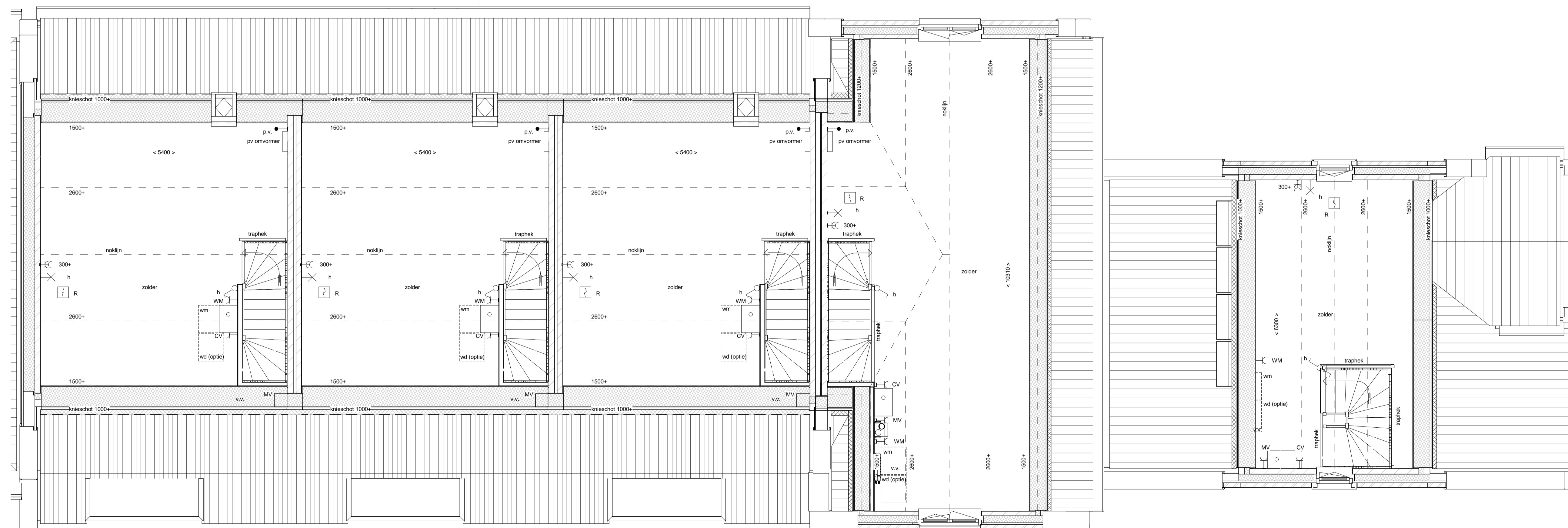
2e Verdieping
