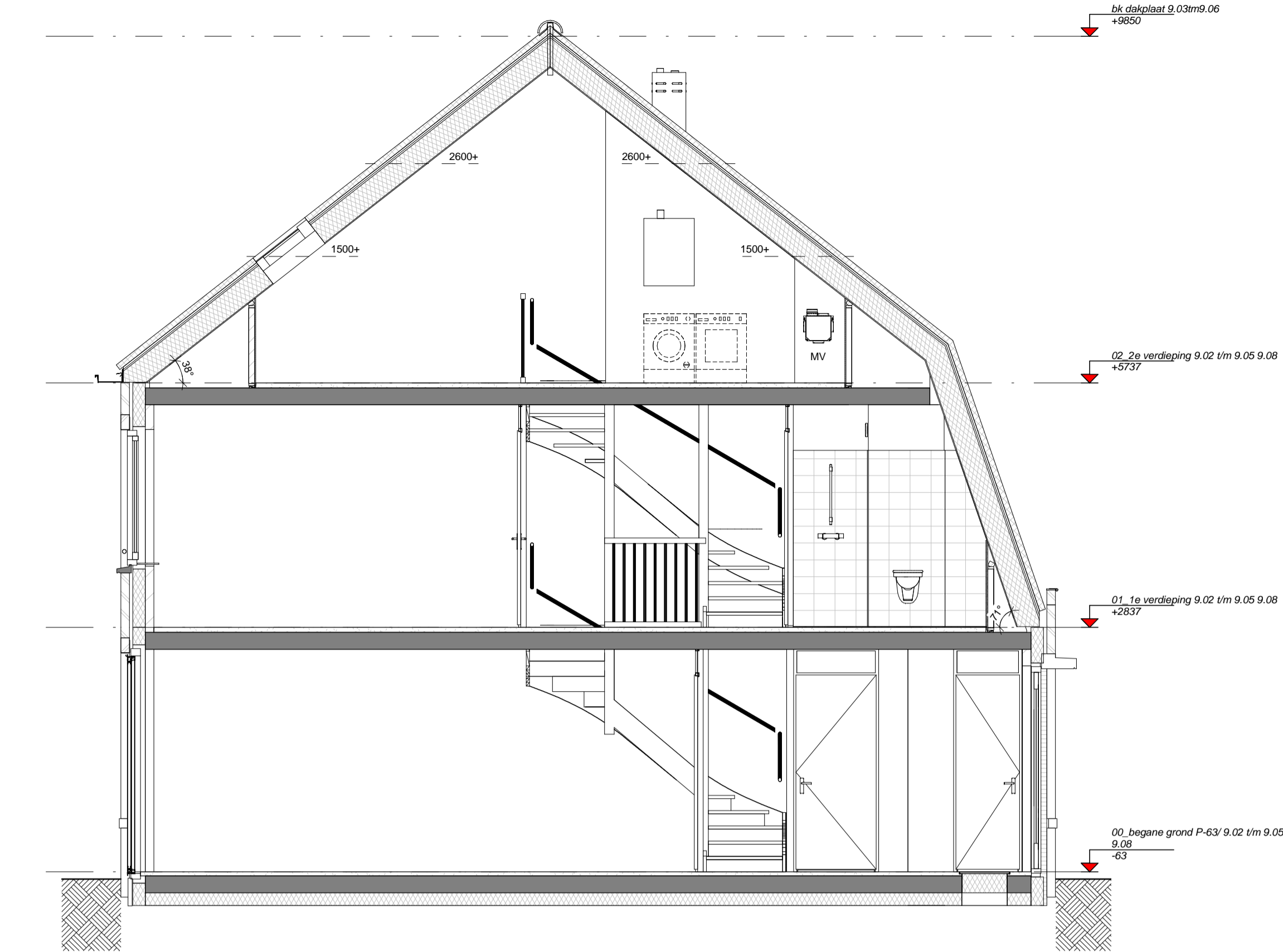
Doorsnede B-B
