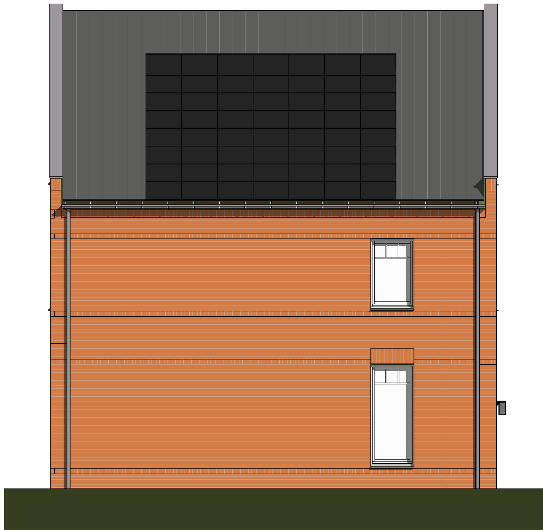
Linker zijgevel
