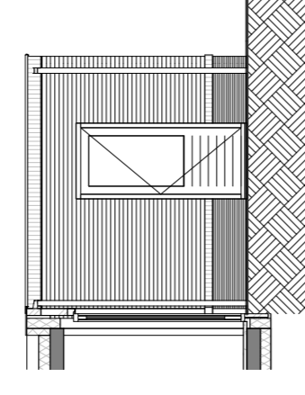
Rechterzijgevel bwnr 67 schaal 1 : 100
