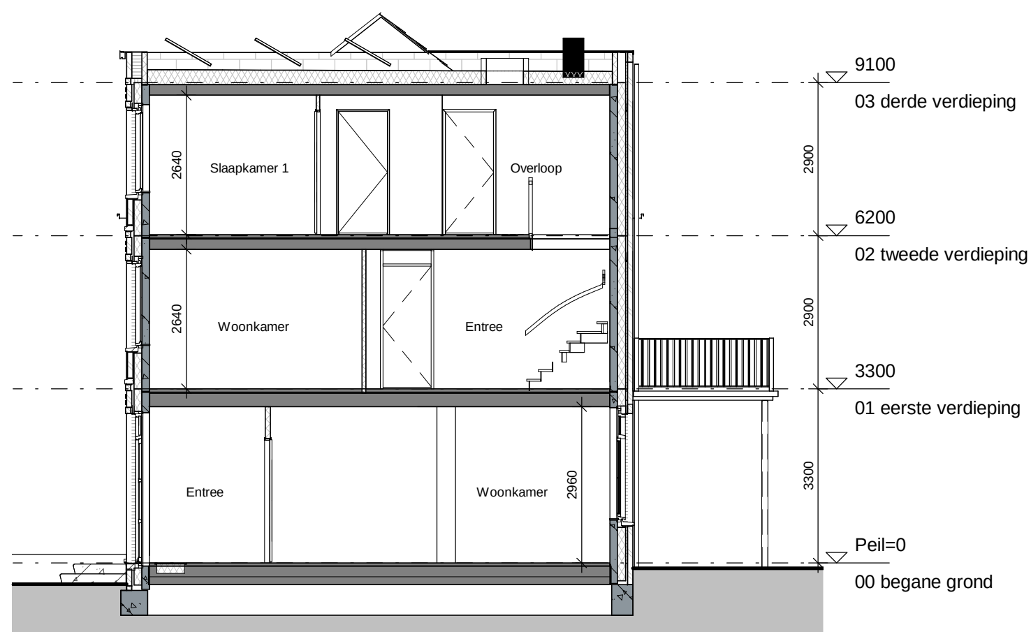
BN112-114 112_boven rechts 111_boven links 114_beneden Doorsnede C
