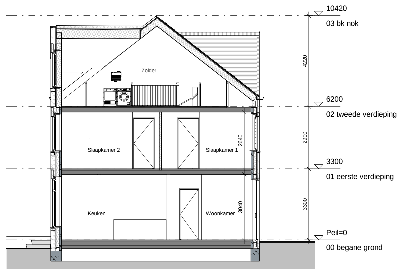
BN108 Doorsnede B
