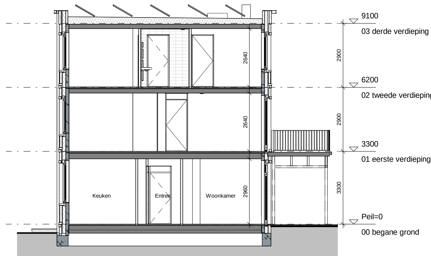
BN101-103 101_beneden 102_boven rechts 103_boven links Doorsnede A
