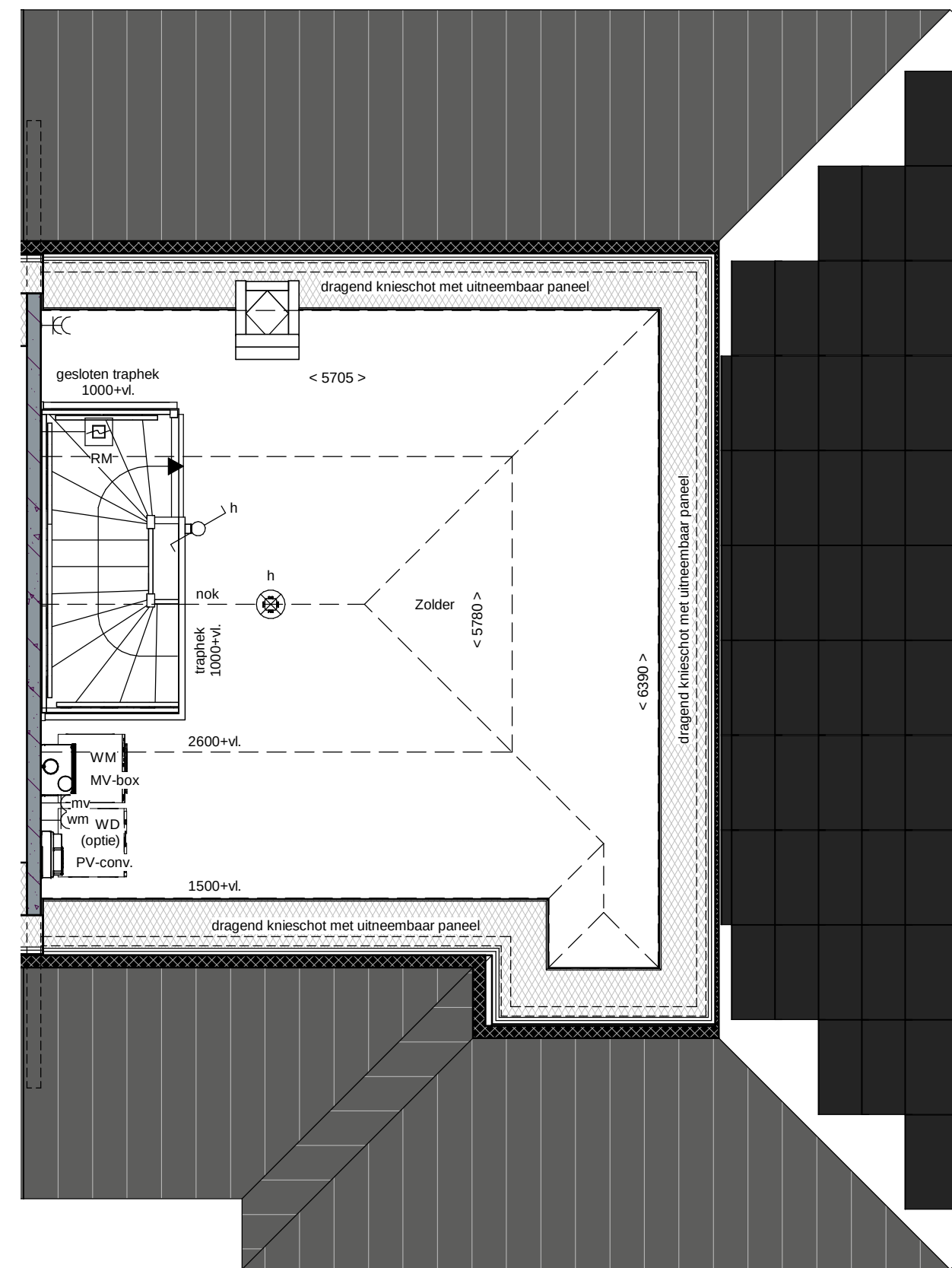
2e Verdieping
