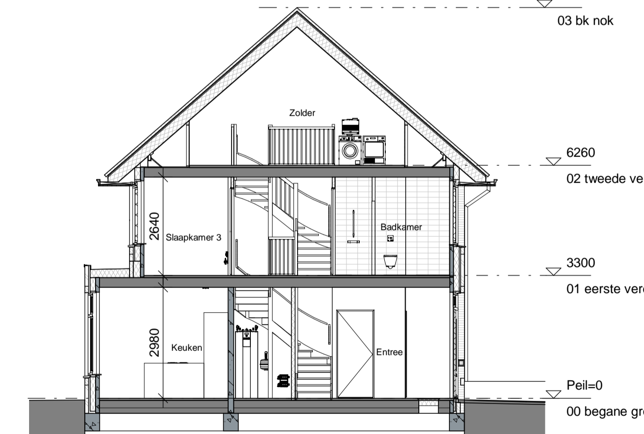
Doorsnede A
