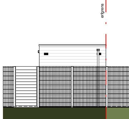
Achtergevel
