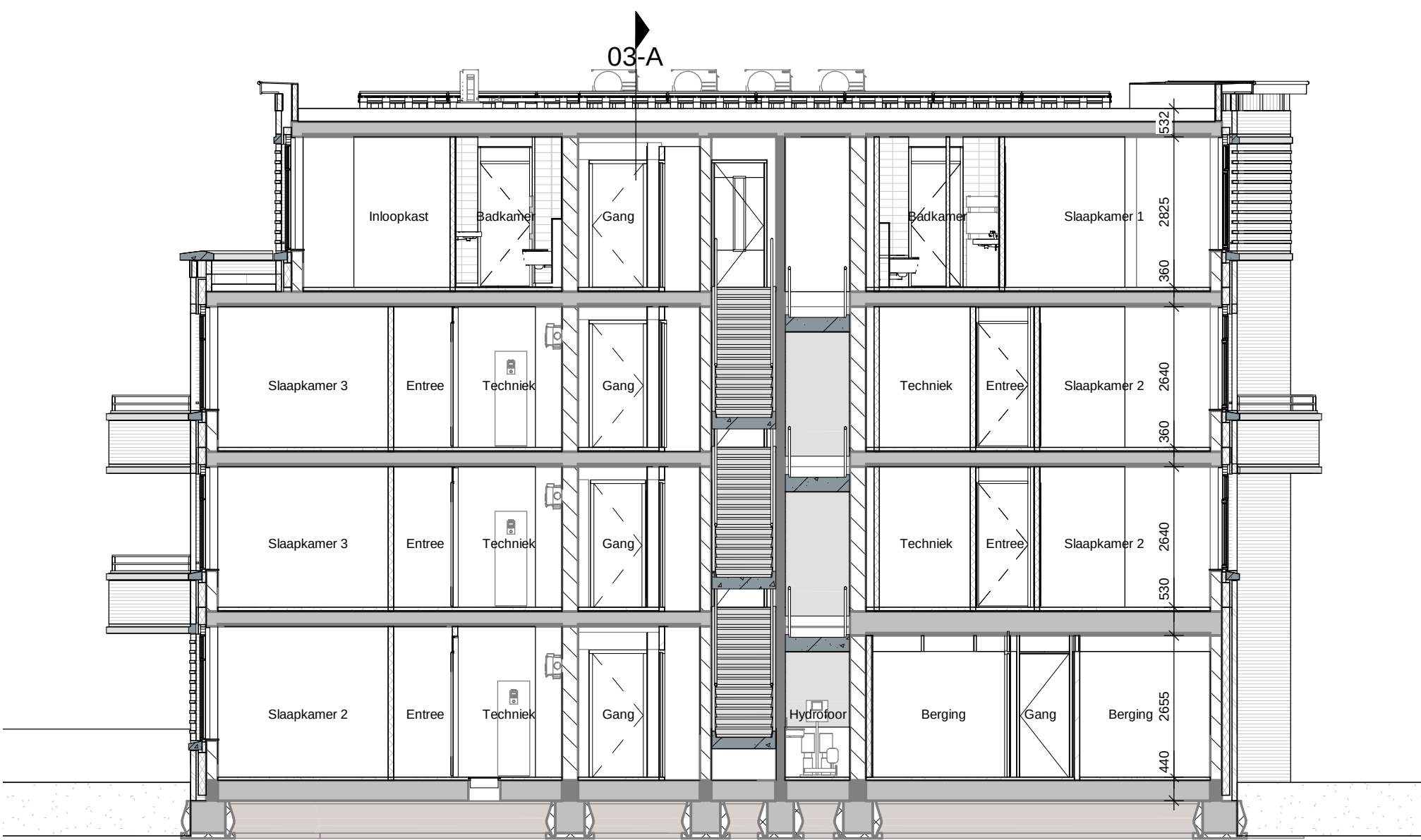
Doorsnede 03-B
