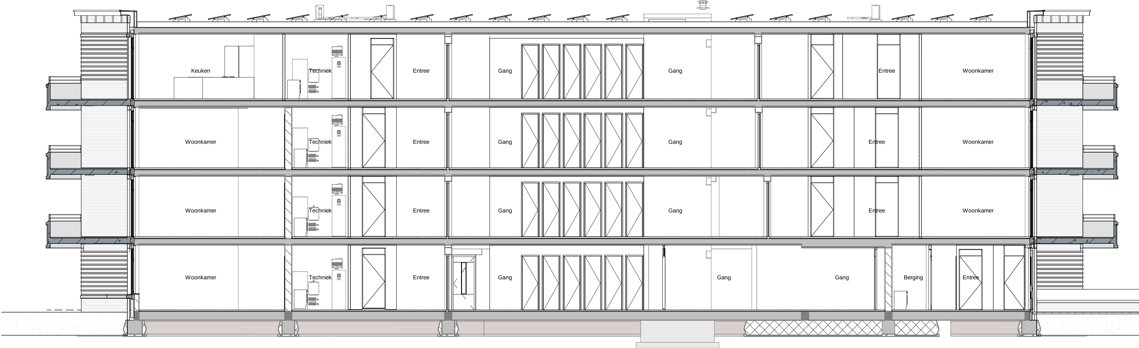
Doorsnede 03-A
