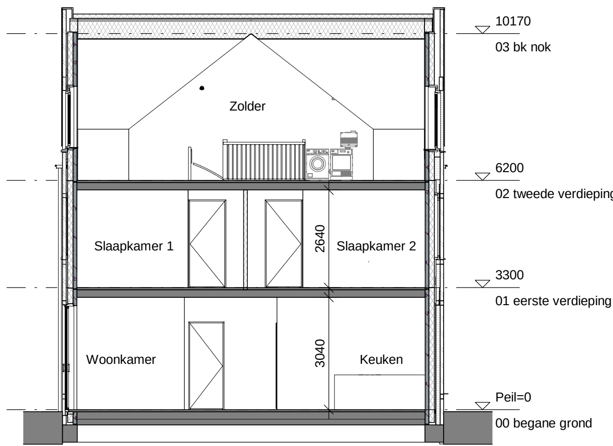
Doorsnede A
