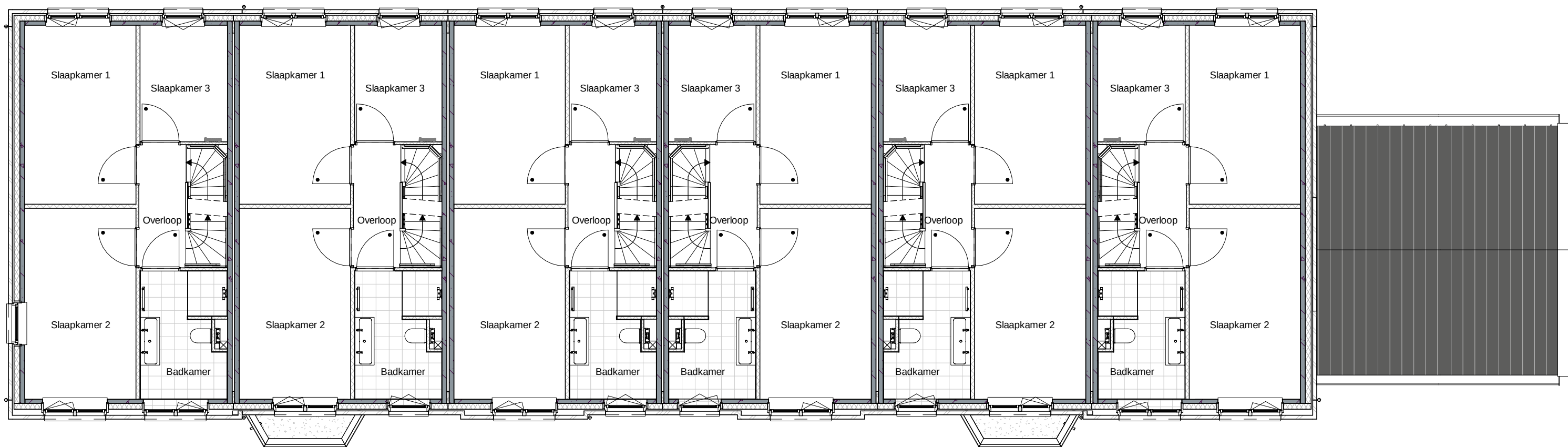
BN360 BN359 BN358 BN357 BN356 BN355 1e Verdieping
