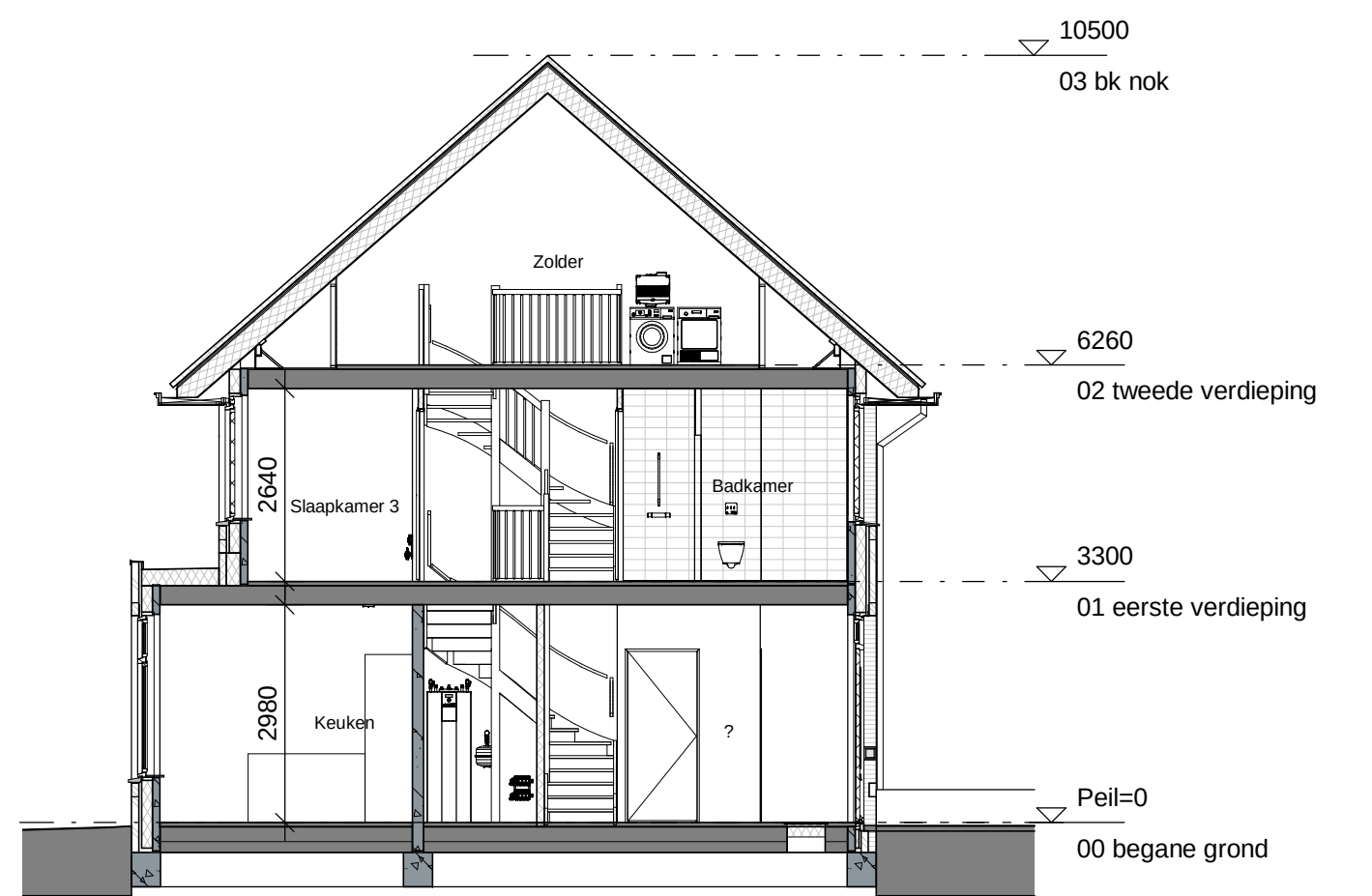
Doorsnede A
